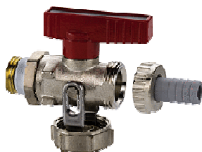
KFE-Kugelhahn PN 16 mit Flügelgriff mit Schlauchverschraubung
